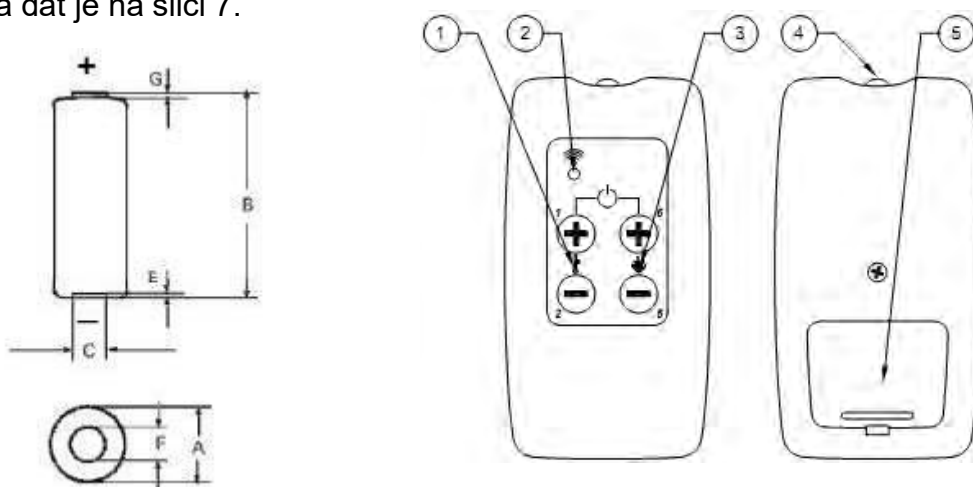
Slika 7. Izgled baterije i daljinskog upravljača (1 - tasteri za podešavanje temperature, 2 - indikator daljinskog upravljača, 3 - tasteri za podešavanje režima rada, 4 - odašiljač, 5 - poklopac baterije)
